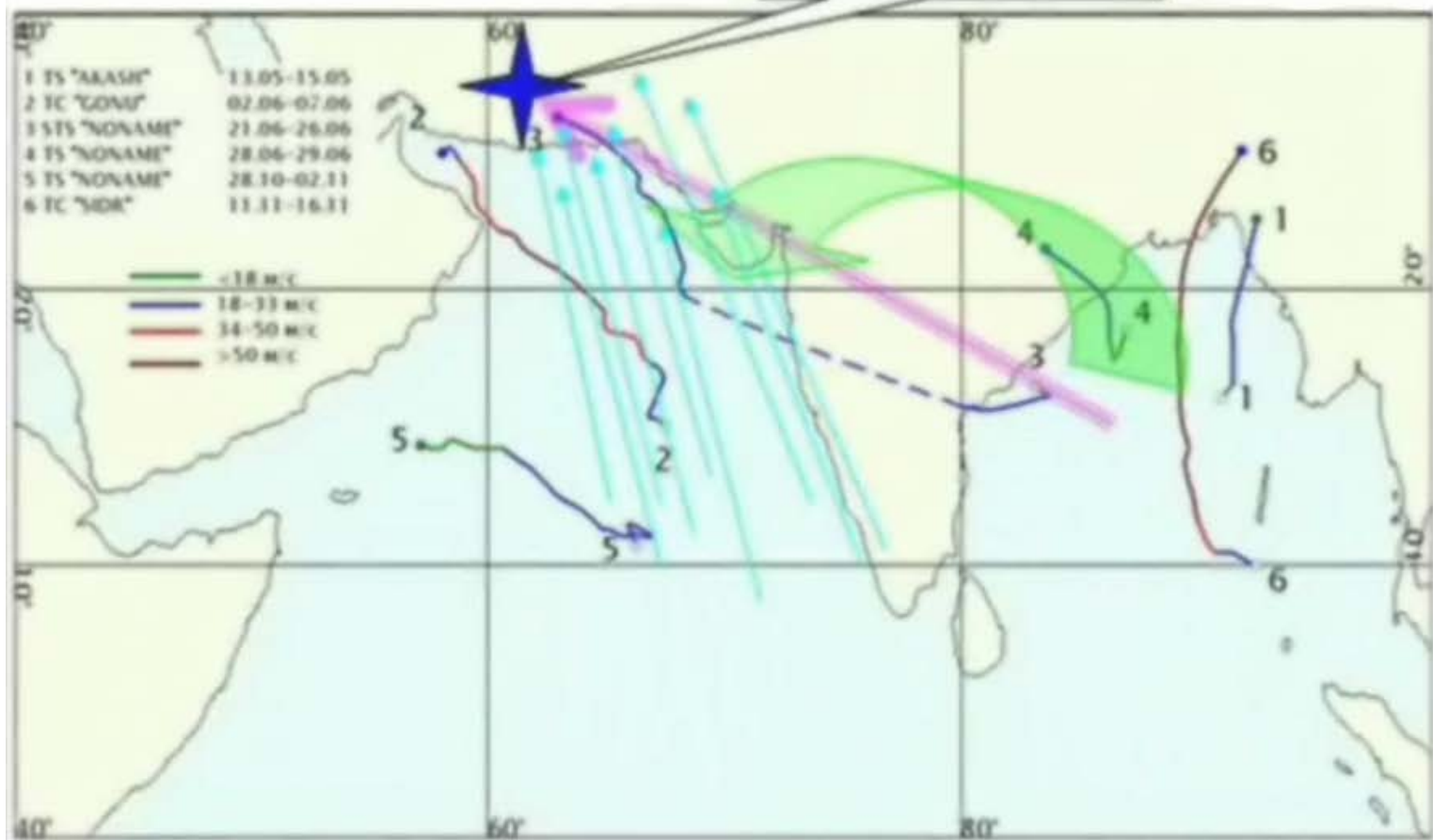
Тропические циклоны северной части Индийского океана в 2007 г.
